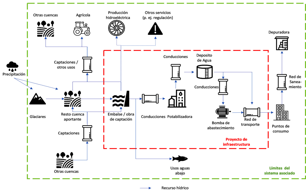
Figura 43: Contexto de evaluación de un proyecto de dotación de agua: propuesta de límites del sistema objeto de estudio
