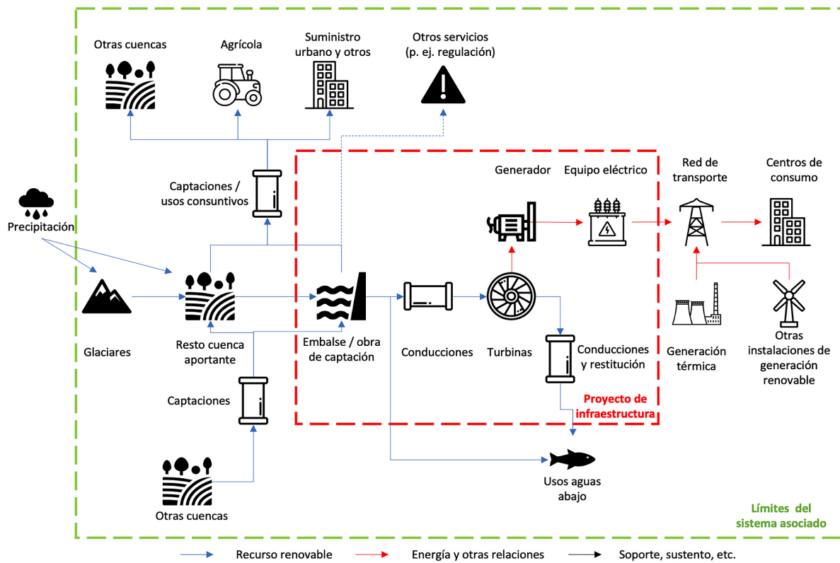
➤ Figura 38: Contexto de evaluación de un proyecto hidroeléctrico: propuesta de límites del sistema objeto de estudio
