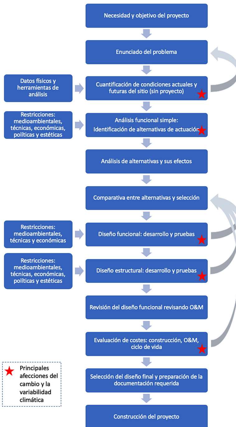
➤ Figura 29: Flujo de diseño general de un proyecto e incorporación de consideraciones de cambio y variabilidad climática
