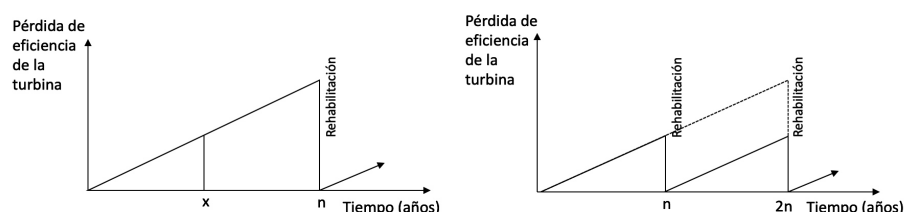
➤ Figura 41: Pérdida de vida útil de la turbina como función del tiempo y de la pérdida de eficiencia (izquierda). Influencia en la planificación de su frecuencia de rehabilitación (derecha)
