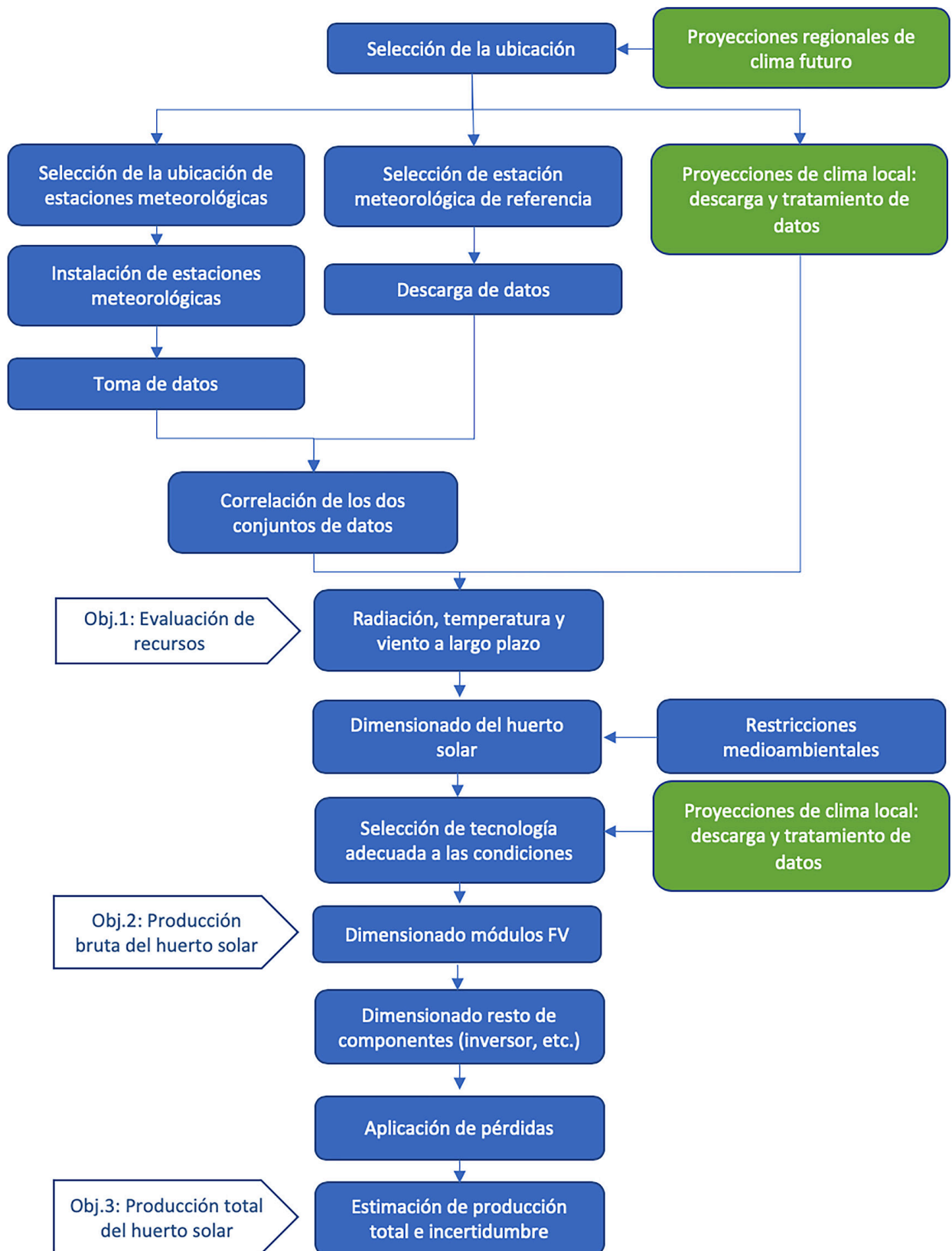
➤ Figura 33: Secuencia metodológica de diseño de un proyecto de infraestructura solar fotovoltaica con consideraciones de clima futuro
