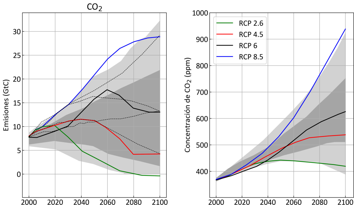
➤ Figura 18: Series temporales de emisiones de gases de efectos invernadero (panel izquierdo) y concentraciones de CO 2 atmosférico (panel derecho) en función de los escenarios RCP
