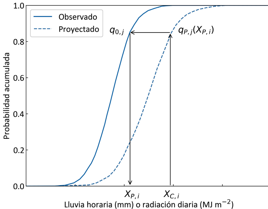
Figura 25: Aplicación del método del mapeo de cuantiles
