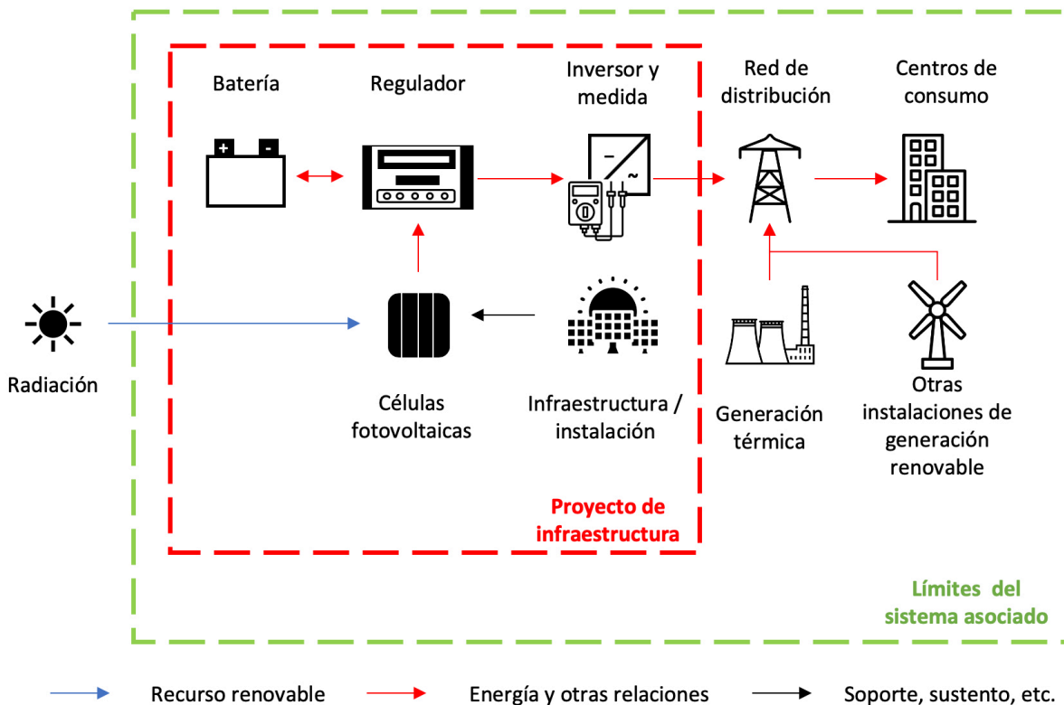
➤ Figura 31: Contexto de evaluación de un proyecto solar fotovoltaico: propuesta de límites del sistema objeto de estudio
