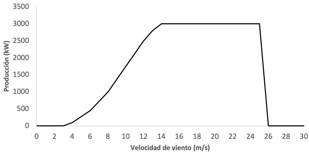
Figura 7: Ejemplo de análisis cuantitativo de la sensibilidad basado en un modelo físico, en el que se establece una relación directa entre una variable climática y el funcionamiento de un proyecto
