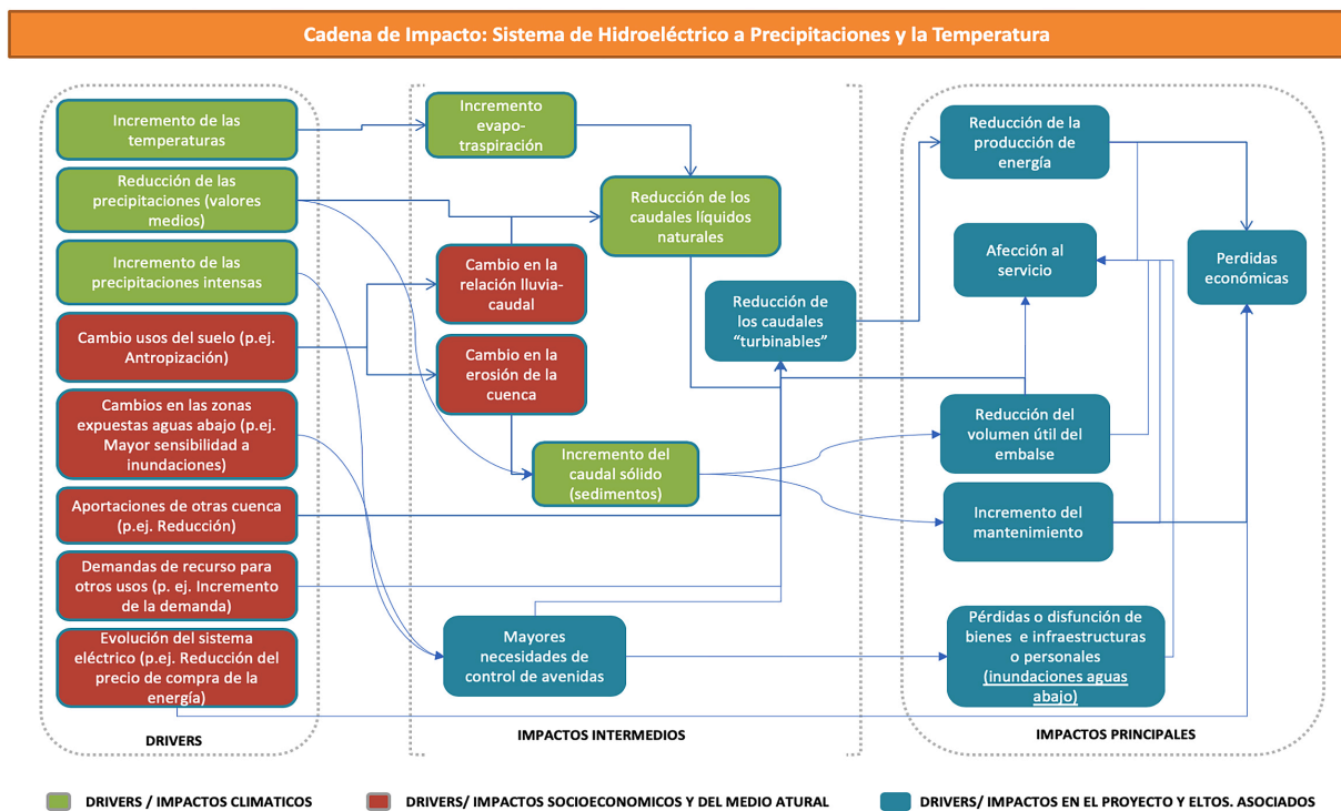
➤ Figura 39: Cadenas de impacto del cambio climático para proyectos hidroeléctricos
