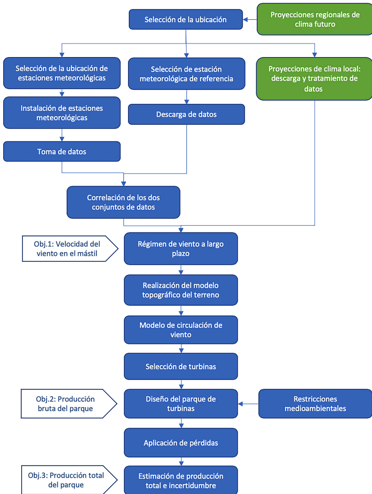
➤ Figura 36: Secuencia metodológica de diseño de un proyecto de infraestructura eólica con consideraciones de clima futuro
