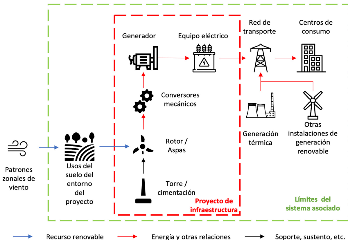
➤ Figura 34: Contexto de evaluación de un proyecto eólico: propuesta de límites del sistema objeto de estudio
