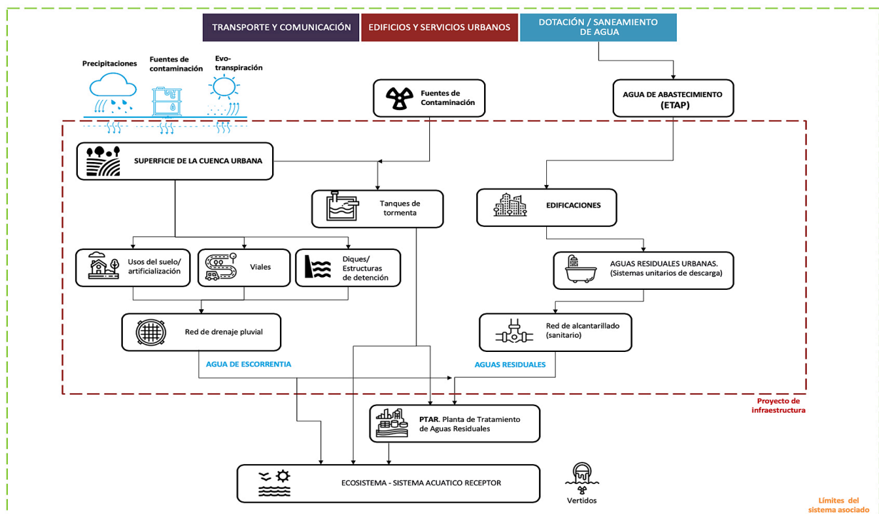
➤ Figura 52: Componentes típicos del sistema de drenaje urbano
