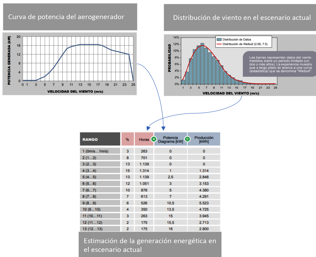
Figura 37: Ejemplo de metodología de cálculo de la producción eólica en un único escenario climático
