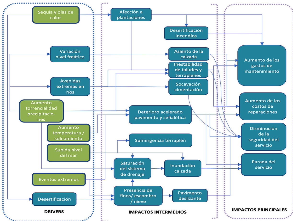
Figura 50: Cadenas de impacto del cambio climático para proyectos de infraestructura vial
