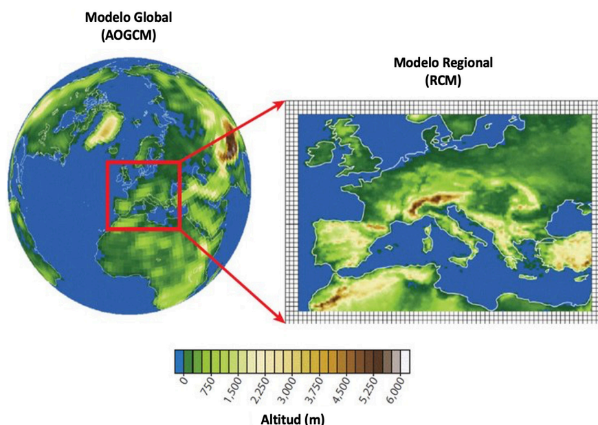
➤ Figura 20: Ejemplo de resolución espacial y dominio de un GCM (izquierda) y de un RCM (derecha)
