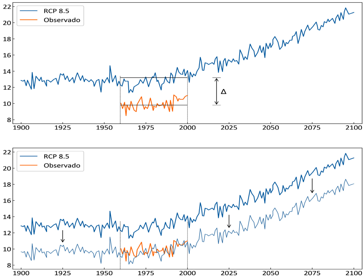
Figura 24: Representación gráfica de la aplicación del método directo a la corrección de sesgo de una serie climática
