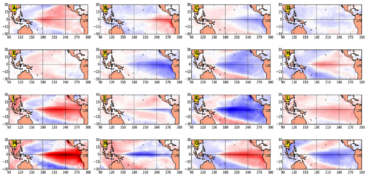
➤ Figura 15: Patrones sinópticos representativos de la anomalía de temperaturas superficiales del mar para la caracterización del fenómeno de El Niño – Oscilación del Sur
