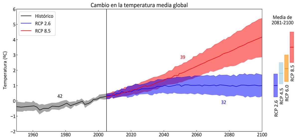
➤ Figura 19: Evolución histórica de la temperatura media global y posibles evoluciones de los diferentes escenarios, con sus valores medios sobre el periodo 2081-2100
