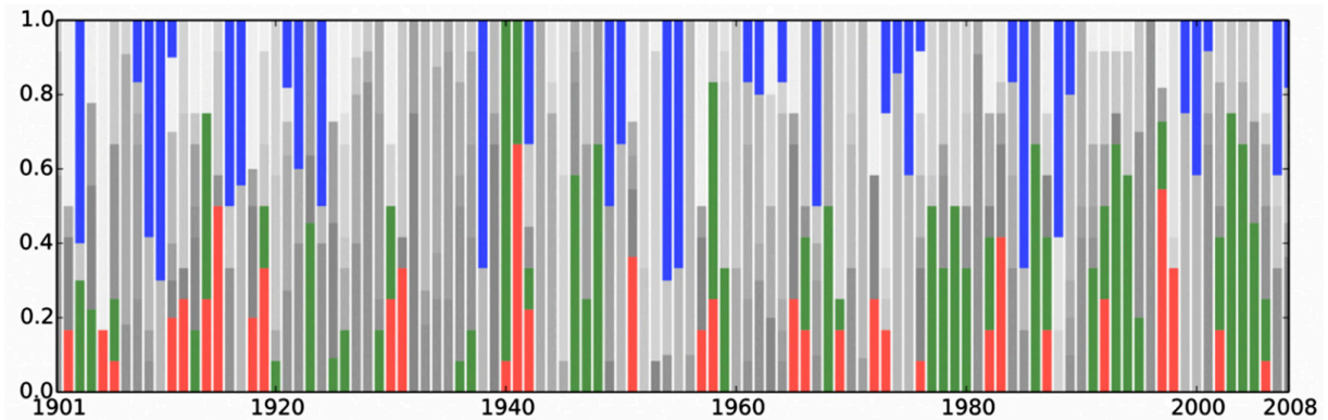
Figura 16: Persistencias (como fracción del año) de patrones de El Niño (en rojo), La Niña (en azul) y el Niño Modoki (en verde)
