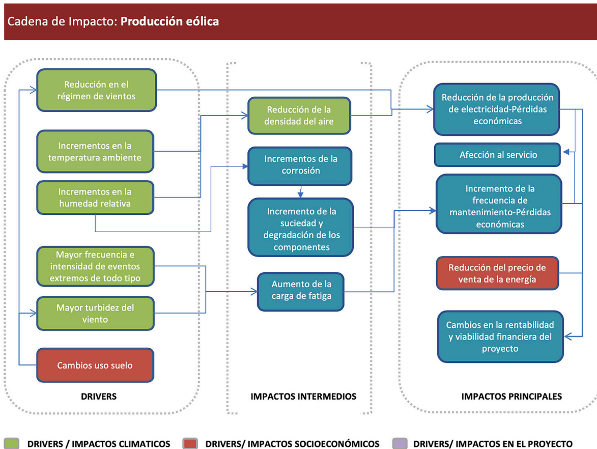
➤ Figura 35: Cadenas de impacto del cambio climático para proyectos eólicos
